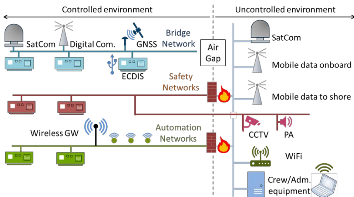
Figur 1 – Generelt datasystem ombord i skip
